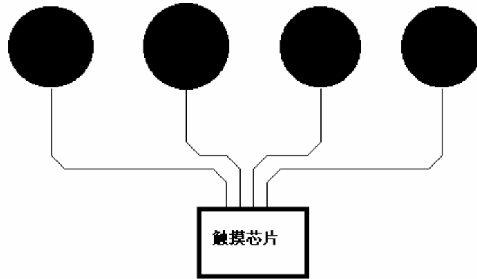
图 2：最好的触摸芯片位置
