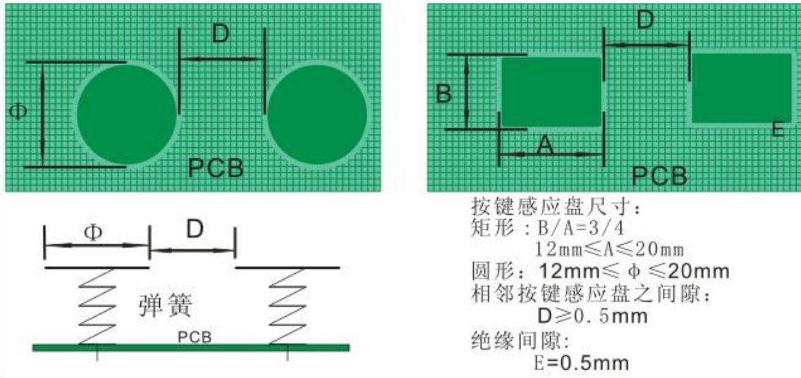
图 4：家电应用中，感应盘大小和间距的推荐尺寸
