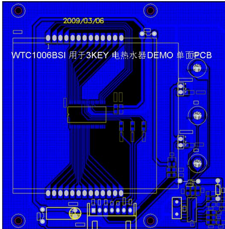
图 12: 采用单面 PCB 板, 弹簧作按键感应盘的 3 键电热水器触控板实例 8.
