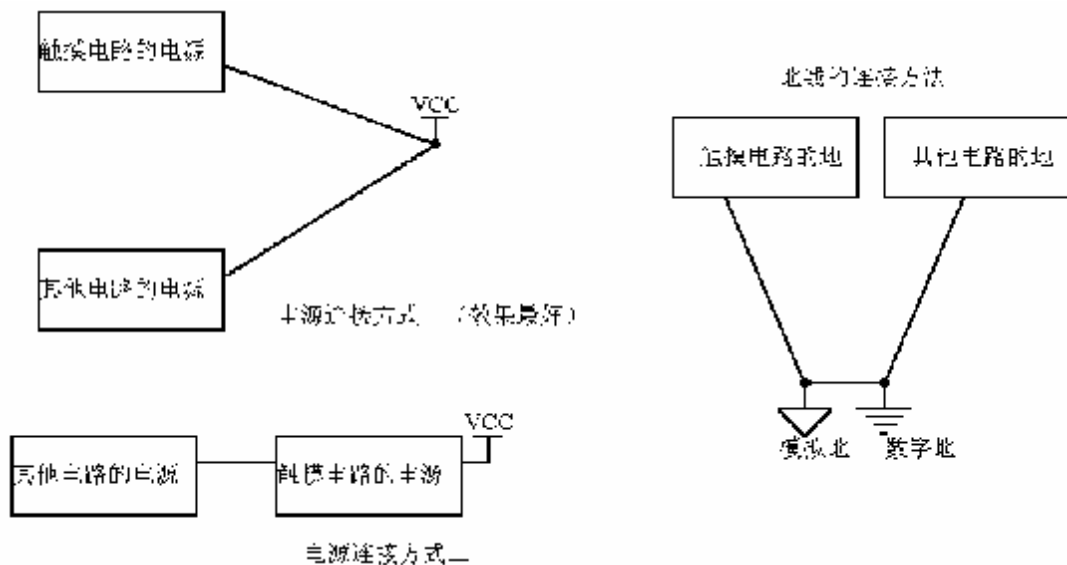
图 1: 电源和地线连接方法示意图
