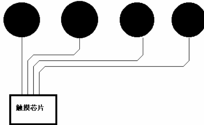
图 3：不好的触摸芯片位置
