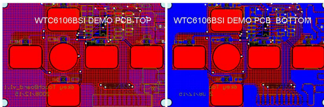
图 11：采用双面板铜箔作按键感应盘 6 键 PCB 板实例
