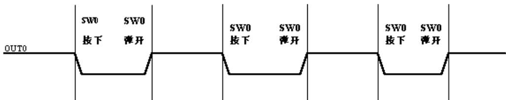
图 2: WTC6106DNI 按键输出时序图
