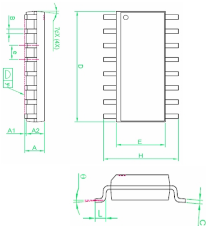
图 8: WTC6106DNI 封装尺寸图
