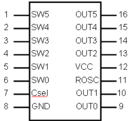
图 1: WTC6106DNI 引脚图
