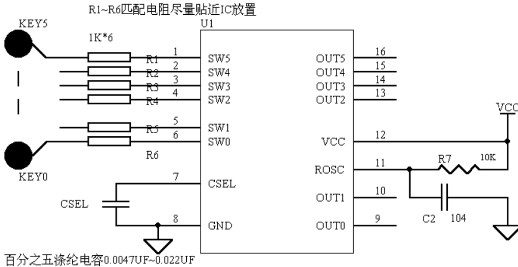
图 3: WTC6106DNI 应用原理图
