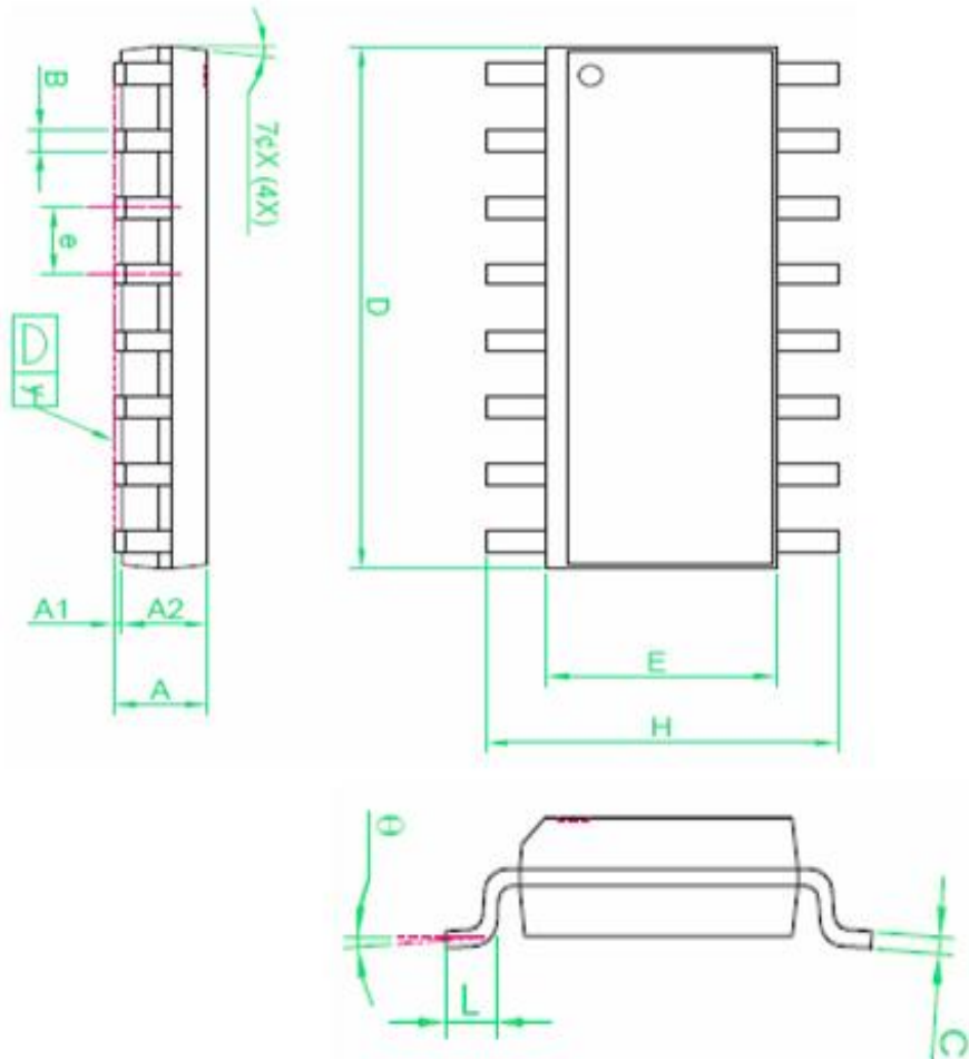
图 8: WTC6106BLV 封装尺寸图
