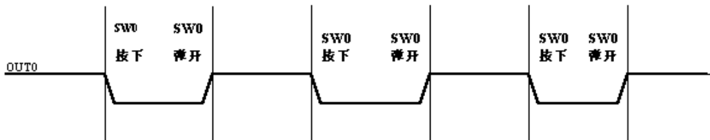
图 2: WTC6106BLV 按键输出时序图
