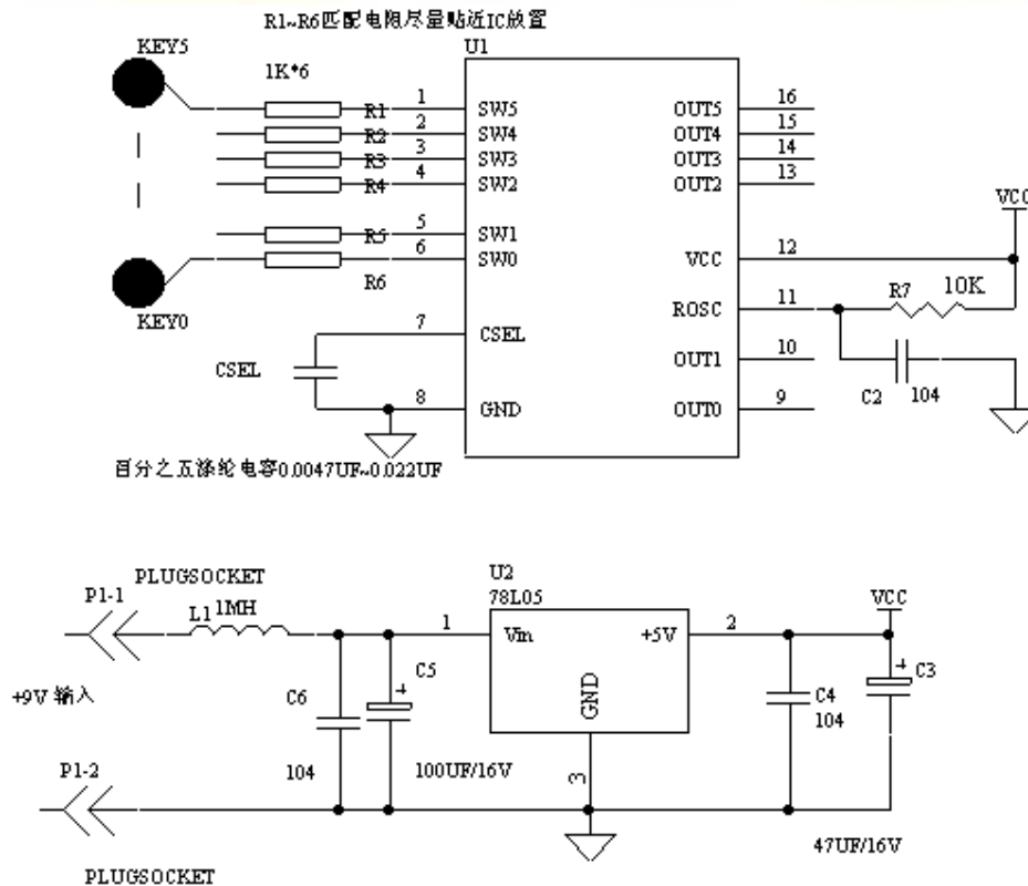
图 4: 电源稳压电路
