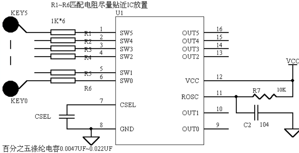
图 3: WTC6106BLV 应用原理图
