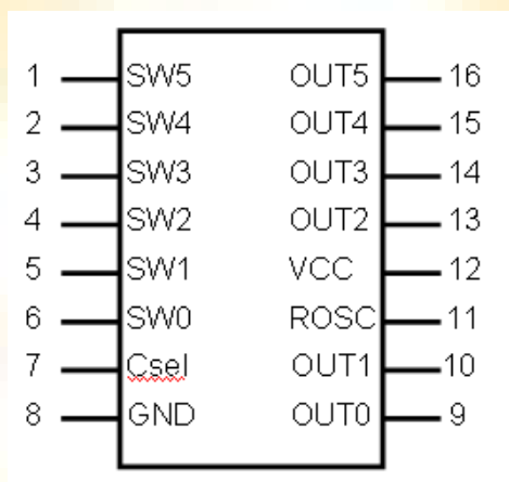
图 1: WTC6106BLV 引脚图
