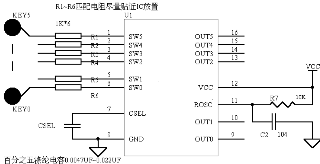
图 3: WTC1006BSF 应用原理图
