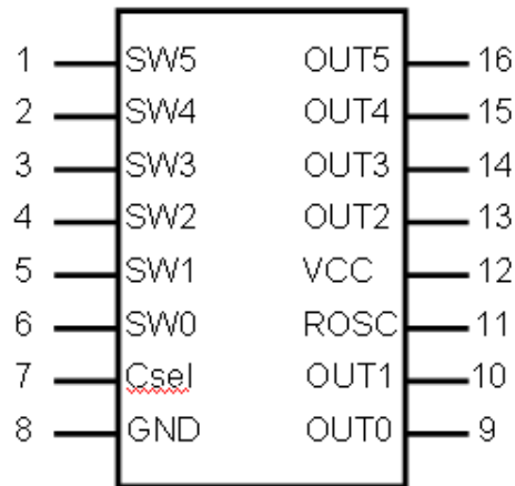
图 1: WTC1006BSF 引脚图
