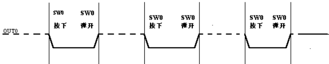
图 2: WTC1006BSF 按键输出时序图
