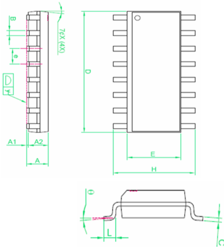
图 8: WTC1006BSF 封装尺寸图
