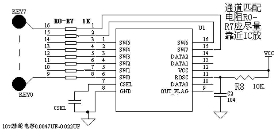
图 3: WTC6208BSI 应用原理图
