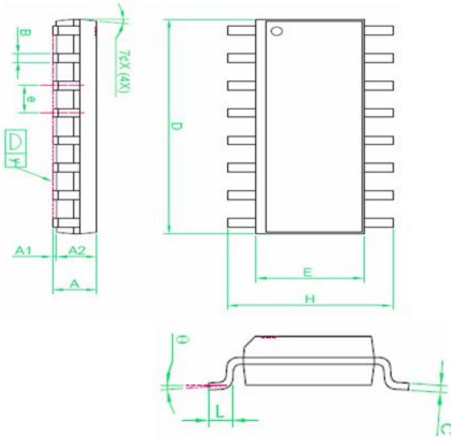
图 8: WTC6208BSI 封装尺寸图
