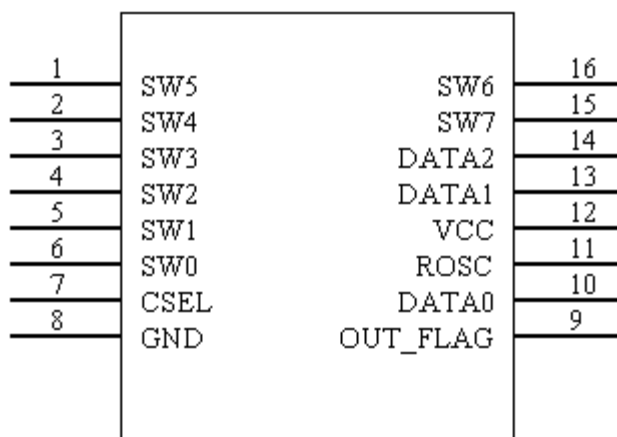
图 1:WTC6208BSI 引脚图
