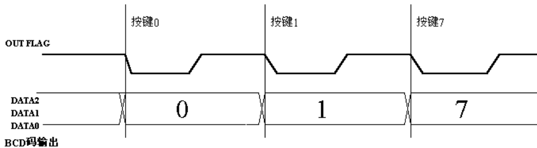
图 2:WTC6208BSI 按键输出时序图
